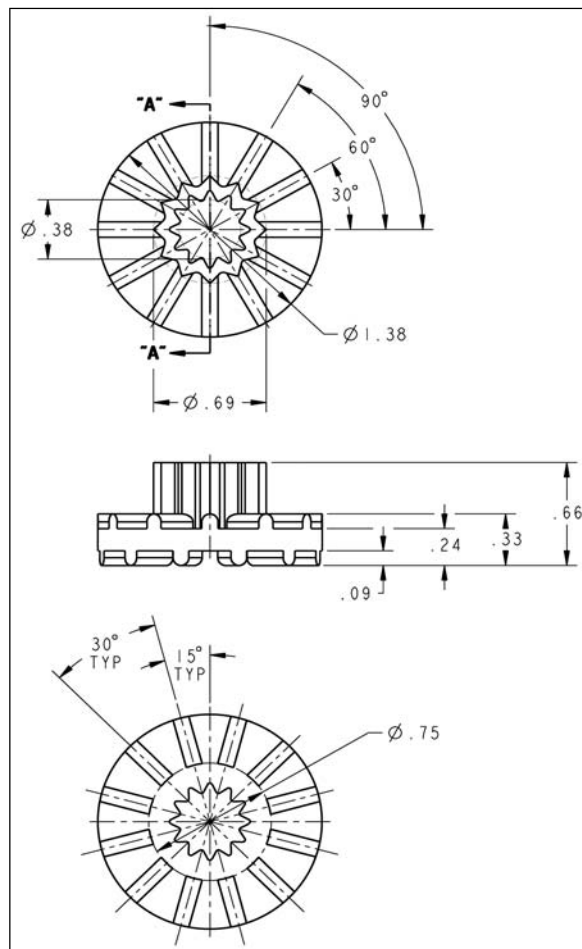
1818 (Bushing)
